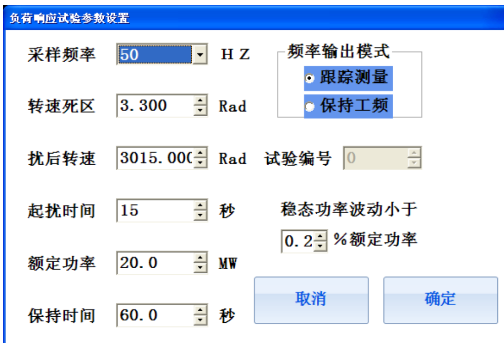
图 16 负荷响应试验参数设置
