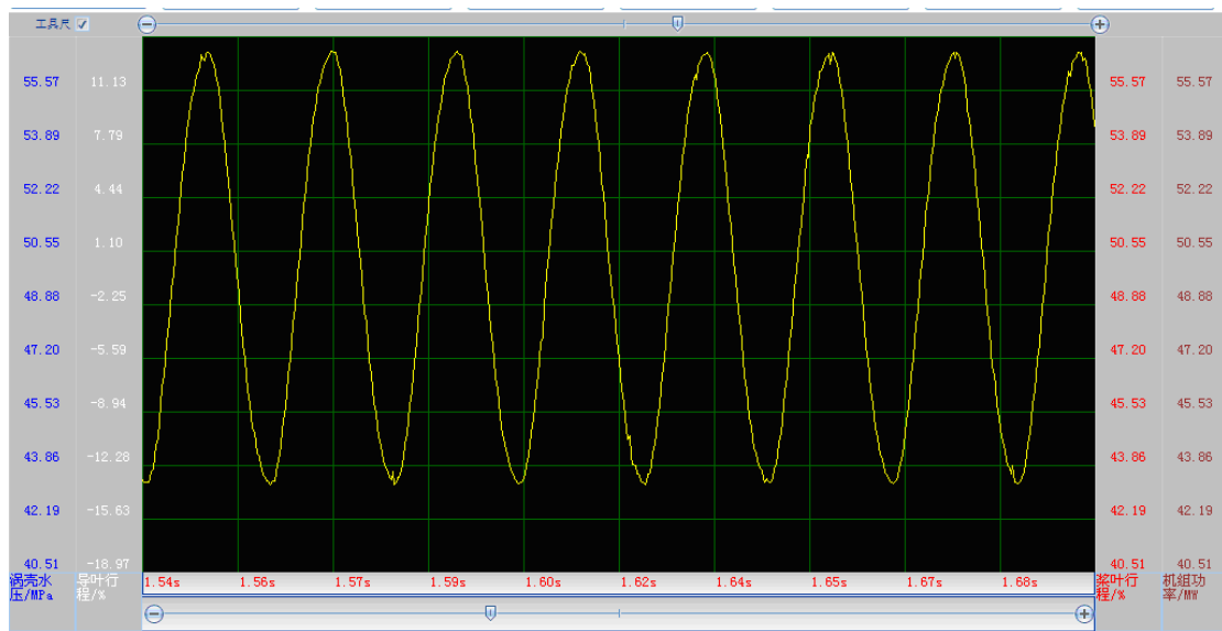
图 21 录波曲线
