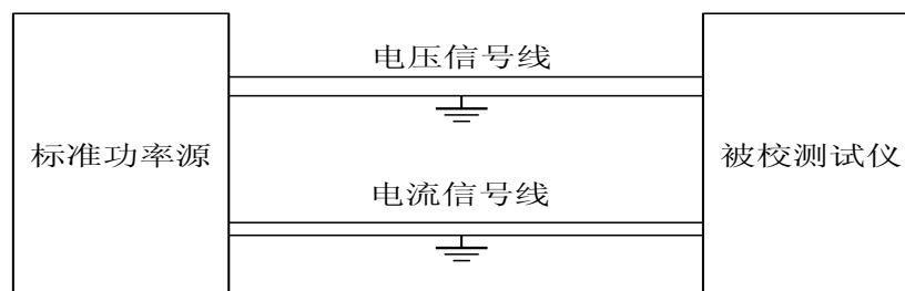
图 2 采用标准波源法校准氧化锌避雷器阻性电流测试仪
