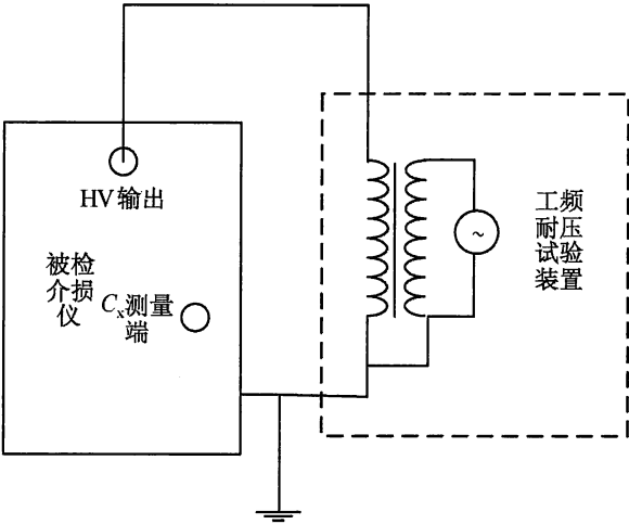
图 2 使用工频耐压试验装置的试验线路
