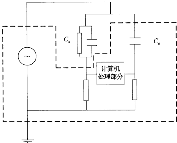
图 1 介损仪工作接线图 C_x —被测电容型设备； C_n —介损仪内置高压标准电容器
